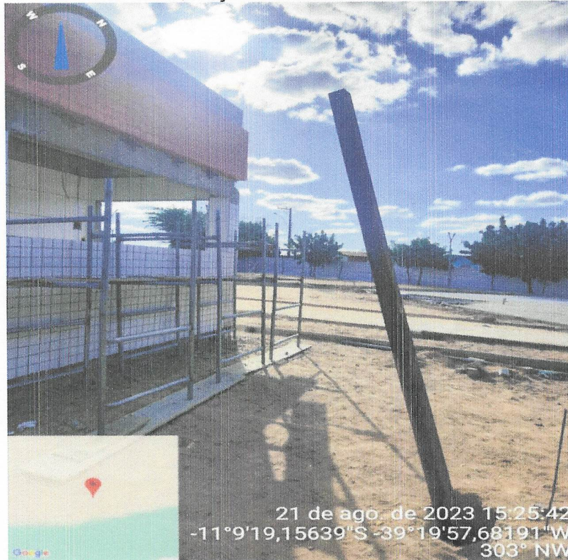
Foto 22- EXECUÇÃO DO PERGOLADO MÉTÁLICO
