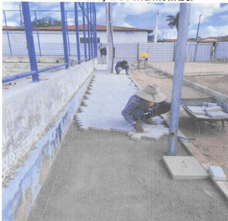
Foto 02 – EXECUÇÃO DO INTERTRAVADO.
