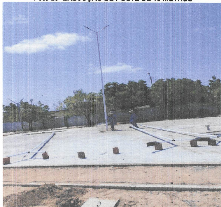
Foto 20- EXECUÇÃO DE POSTE DE 10 METROS
